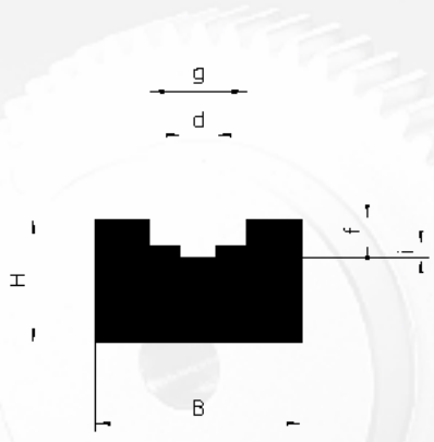
GL 1b zweiteilig 2-parts
