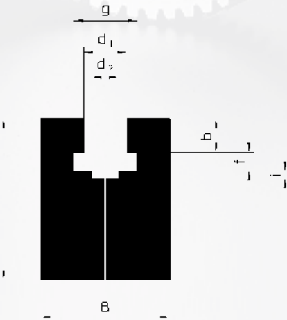
GL 1b zweiteilig 2-parts
